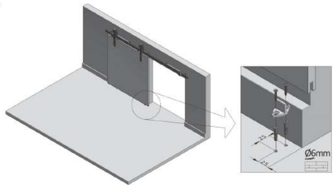
установка флажка
