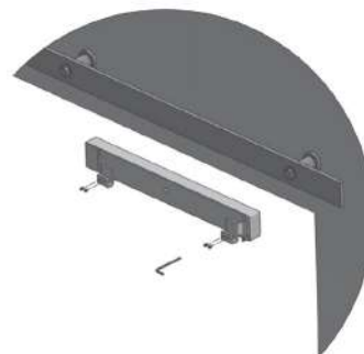
Установка доводчика
